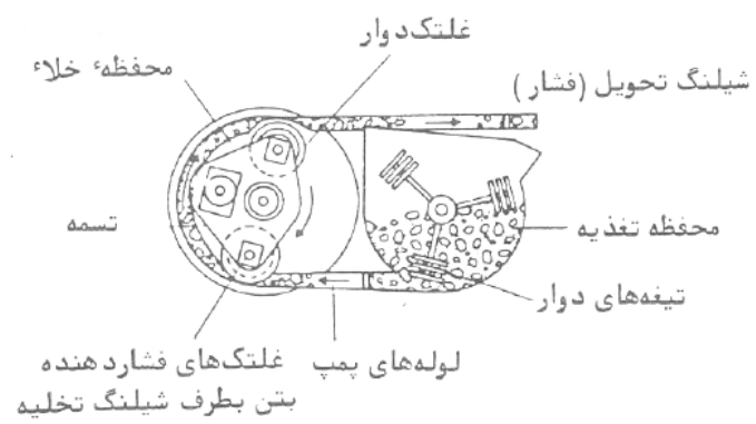
قسمتهای اصلی پمپ بتن
